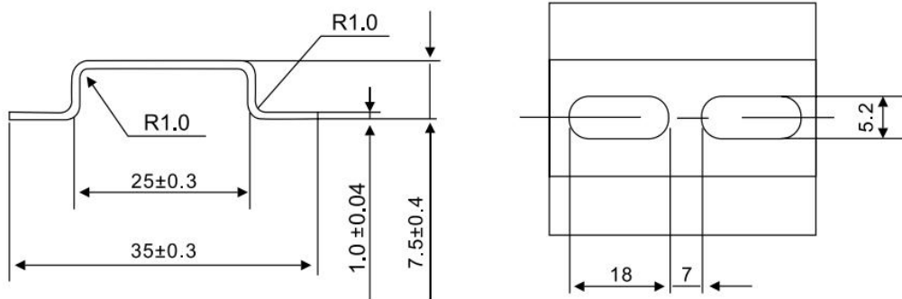
Рисунок 1-1 -DIN-рейка. Общий вид.
